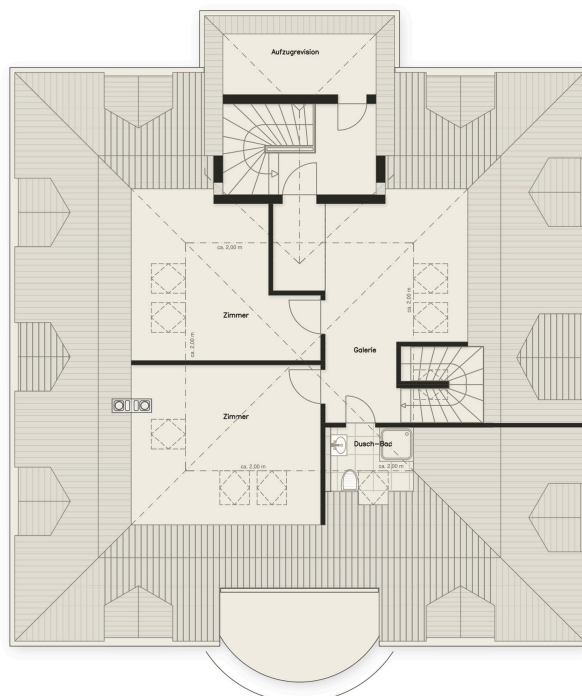
2. DACHGESCHOSS
